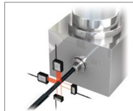
Medición de diámetro exterior/ deformación en la extrusión
