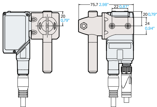
■ Con soporte ajustable (OP-88697)
