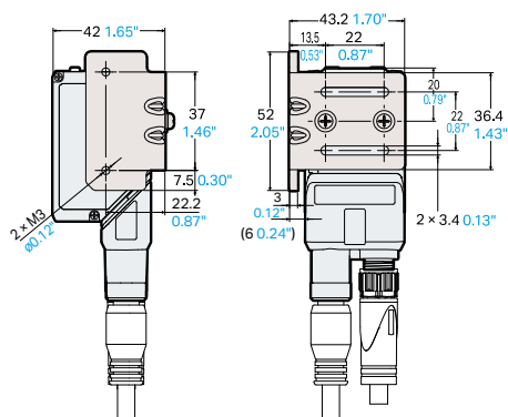
■ Con soporte de montaje intercambiable 1 (OP-88698)
