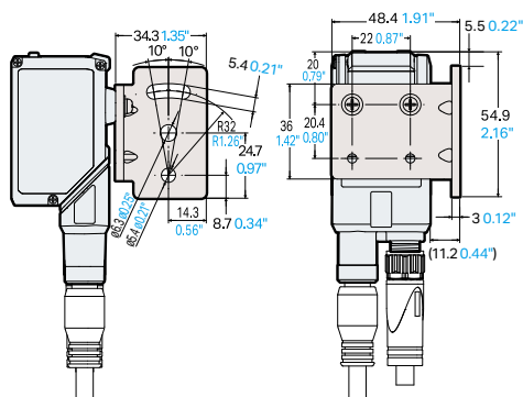
■ Con soporte de montaje intercambiable 2 (OP-88699)
