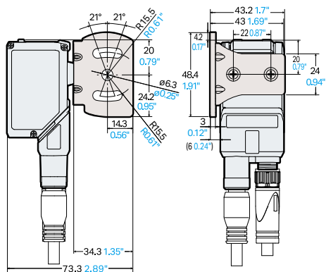
■ Con soporte de montaje (OP-88696)
