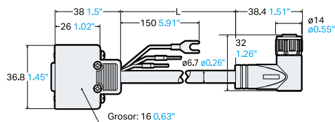
■ Cable Ethernet con conector en forma de L (OP-88301 a OP-88303)
